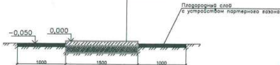
Сечение 3-3 М 1:85
