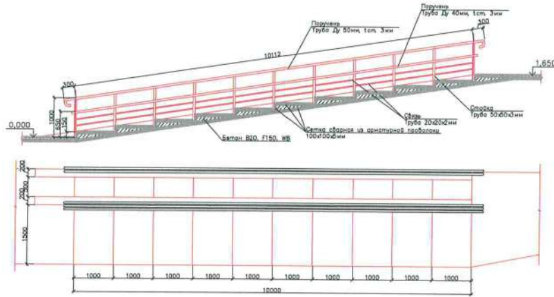
Сечение 1-1 М 1:85
