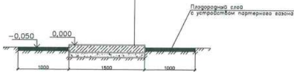
Сечение 3-3 М 1:85
