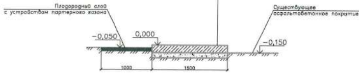
Сечение 2-2 М 1:85
